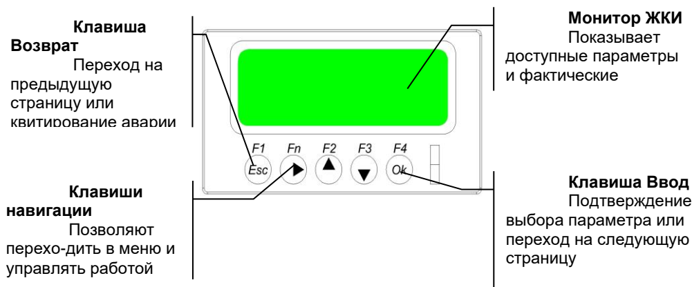
Рисунок 1 - Общий вид управляющего контроллера PIXEL
