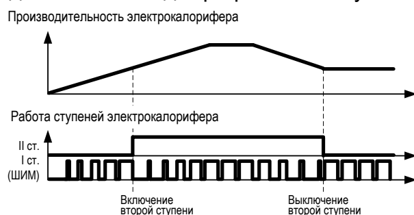
Рисунок 13 – Диаграмма работы электрокалорифера
