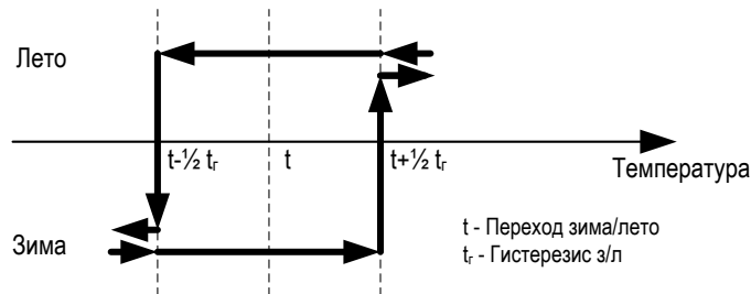
Рисунок 2 – Гистерезис перехода «зима»-«лето»
